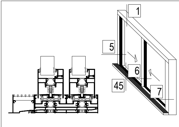
19 Two-sash sliding window with gutter Δίφυλλο επάλληλο συρόμενο με υδατολεκάνη
