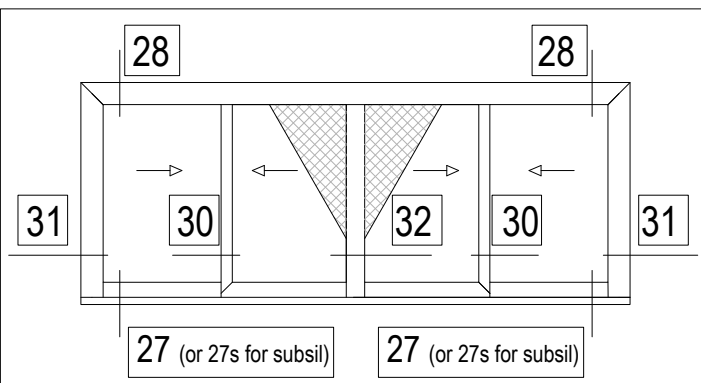
11 Four-sash meeting stile sliding window with flyscreen Τετράφυλλο φιλητό συρόμενο με σήτα
