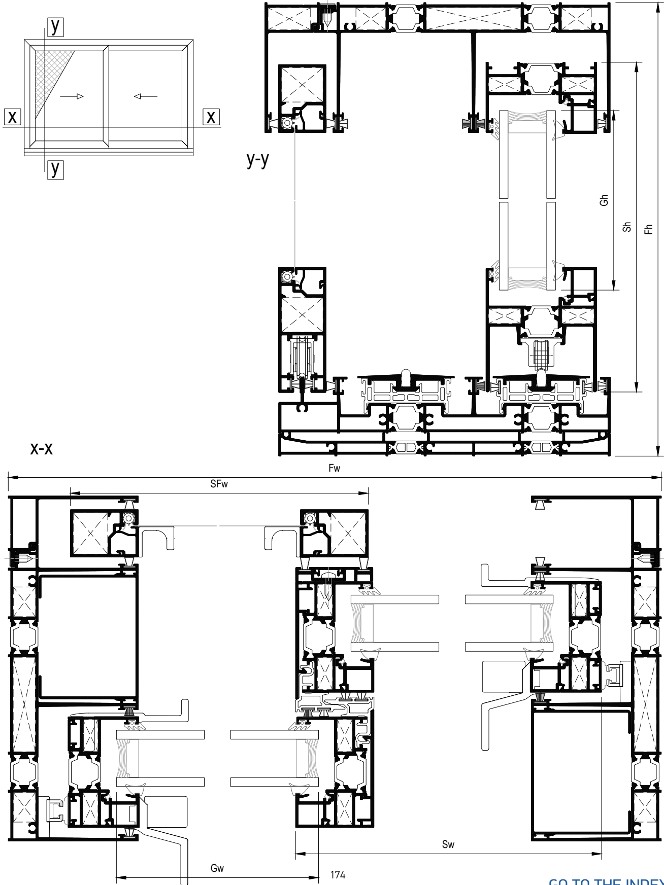
10 Two-sash sliding window with subsil and flyscreen Δίφυλλο επάλληλο συρόμενο με υπόκασα και σήτα
