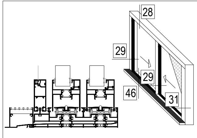
20 Two-sash sliding window with flyscreen and gutter Δίφυλλο επάλληλο συρόμενο με σήτα και υδατολεκάνη
