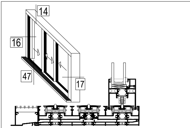
21 Three-sash sliding window with gutter Τρίφυλλο επάλληλο συρόμενο με υδατολεκάνη
