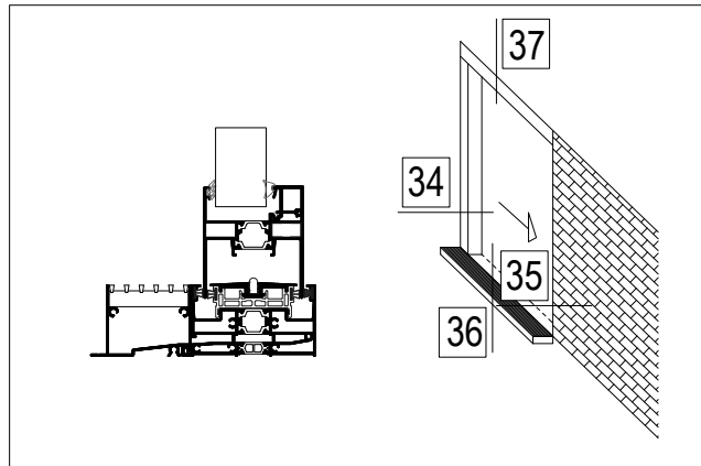
22 One sash pocket window with gutter Μονόφυλλο χωνευτό με υδατολεκάνη
