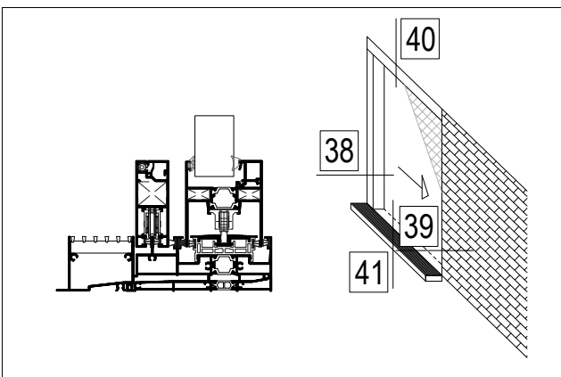
23 One sash pocket window with flyscreen and gutter Μονόφυλλο χωνευτό με σήτα και υδατολεκάνη
