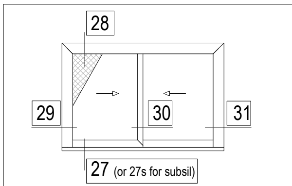
9 Two-sash sliding window with flyscreen Δίφυλλο επάλληλο συρόμενο με σήτα
