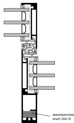
I=114,1 cm 4
